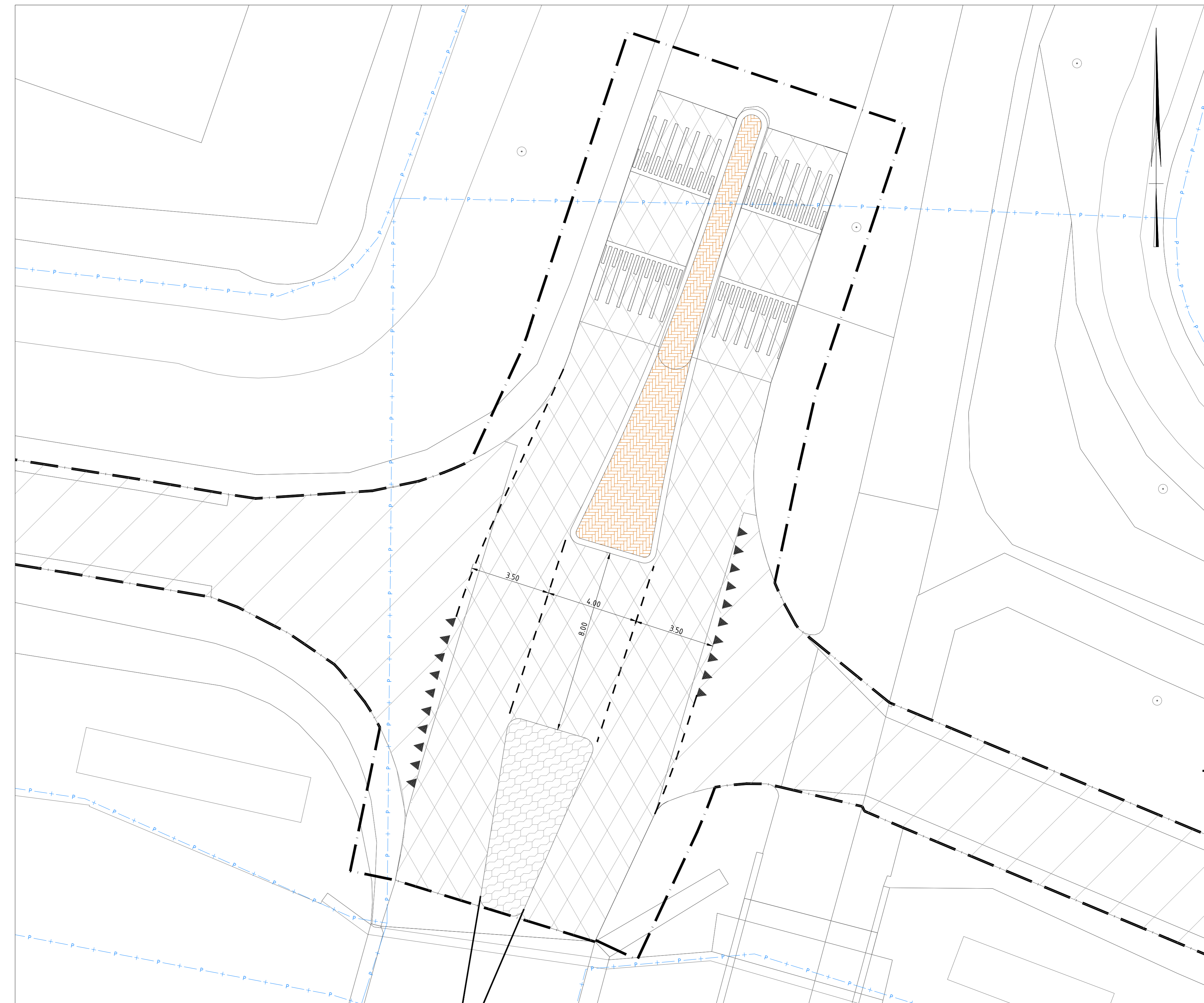
Kruispunt Zandweg - Europaweg, De Meern, schaal 1:100
