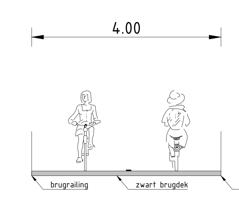
Tweerichtingsverkeer fietspad wegvak 31
