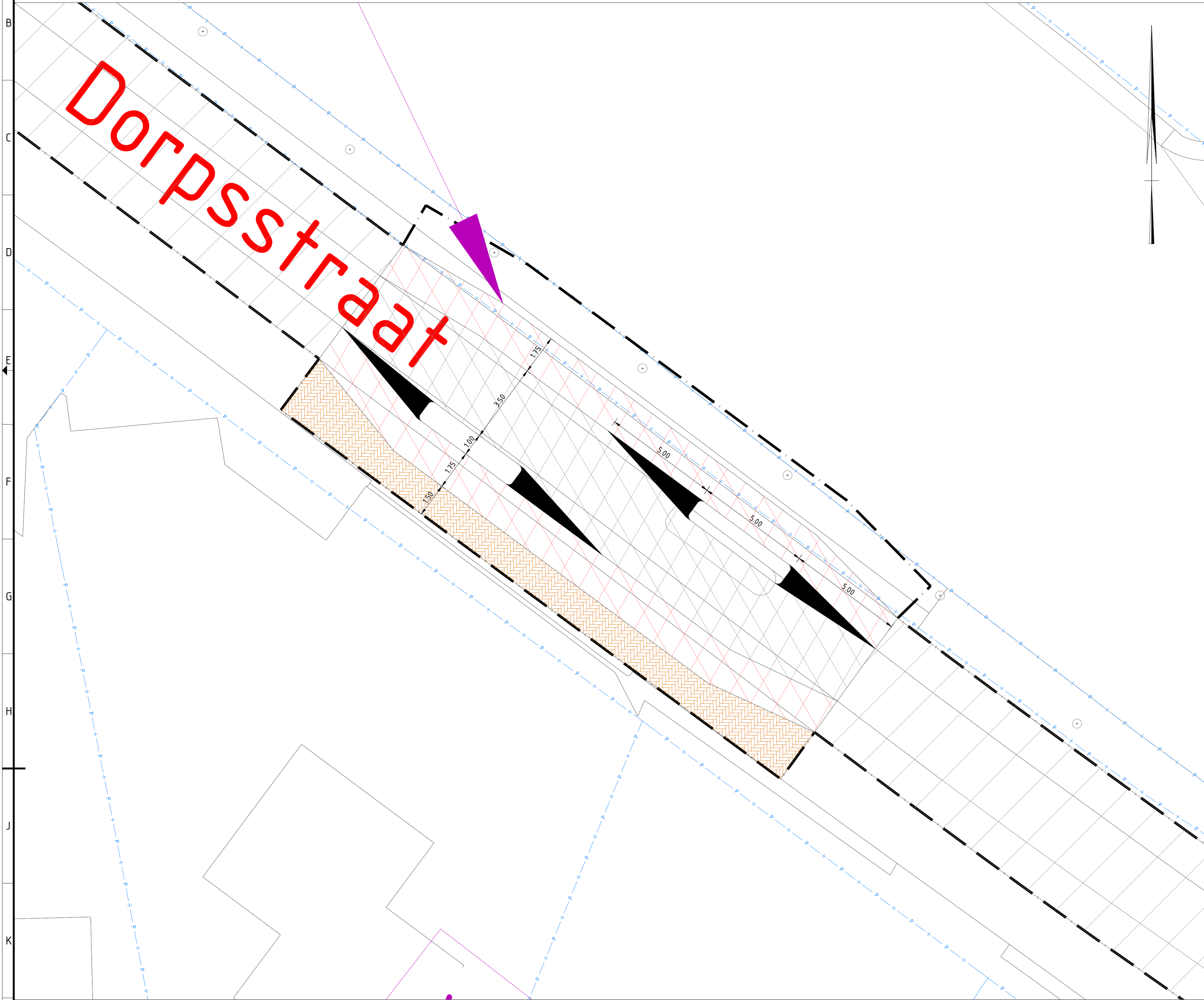
Snelheidsremmer, Dorpsstraat Harmelen, schaal 1:100
