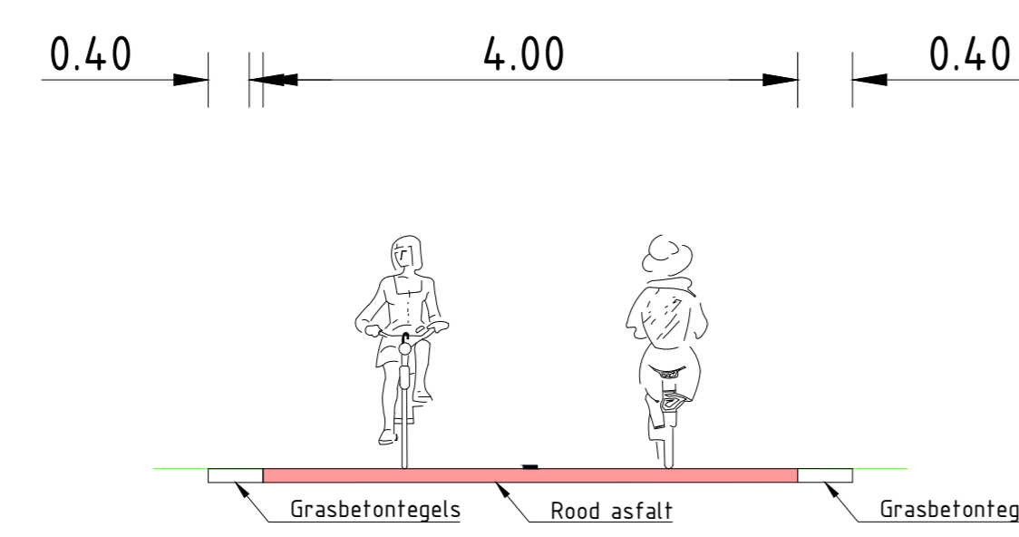
Tweerichtingsverkeer fietspad wegvak 2
