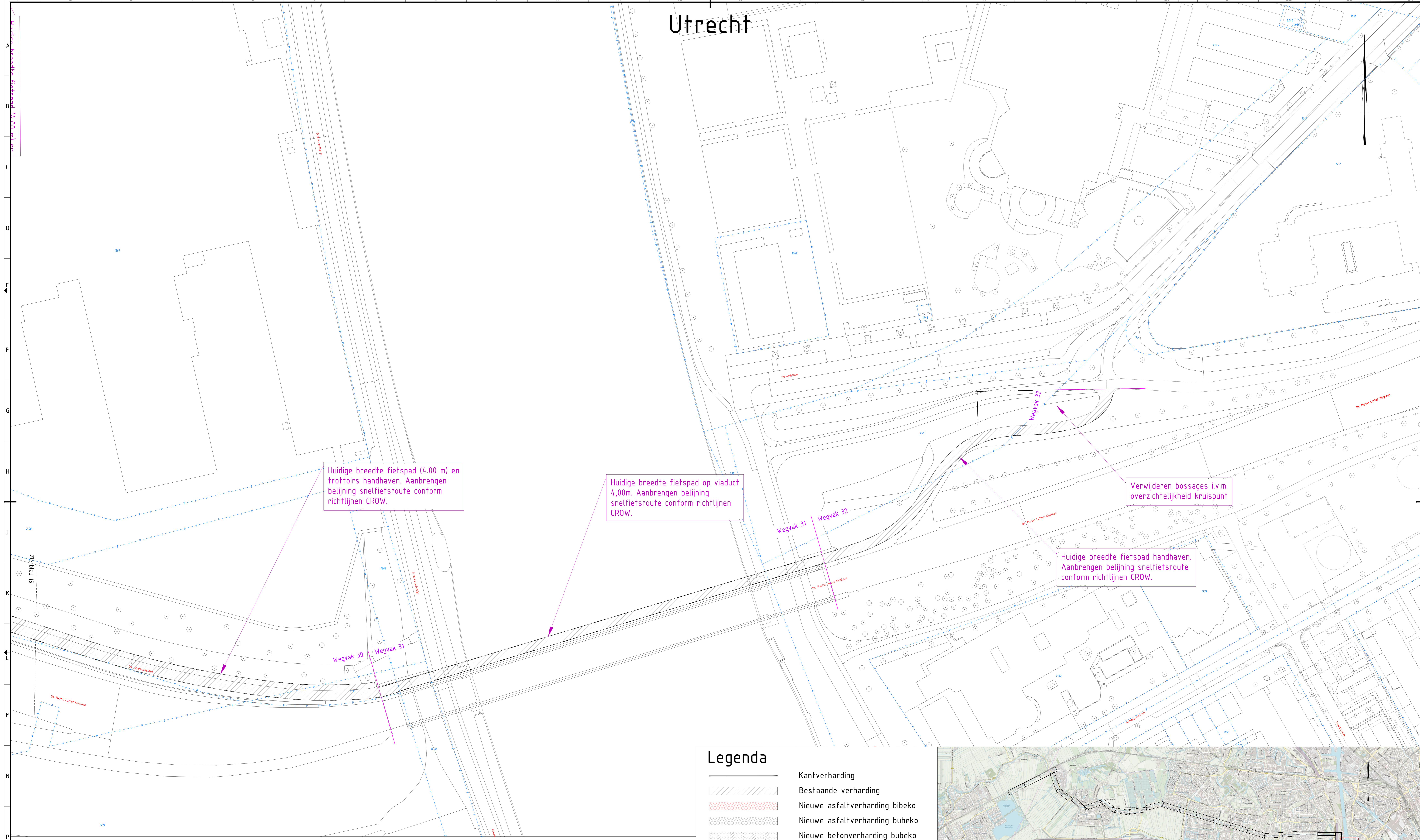
Tweerichtingsverkeer fietspad wegvak 31
