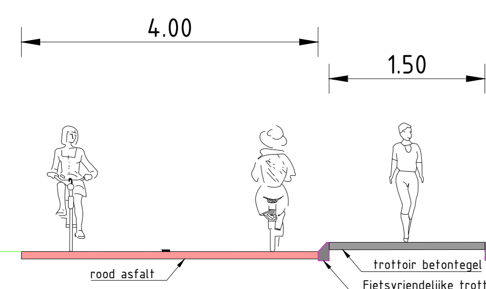
Tweerichtingsverkeer fietspad wegvak 1
