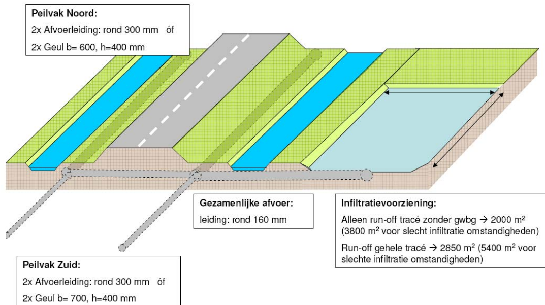
Oplossing 7: Infiltratie via een centrale infiltratievoorziening
