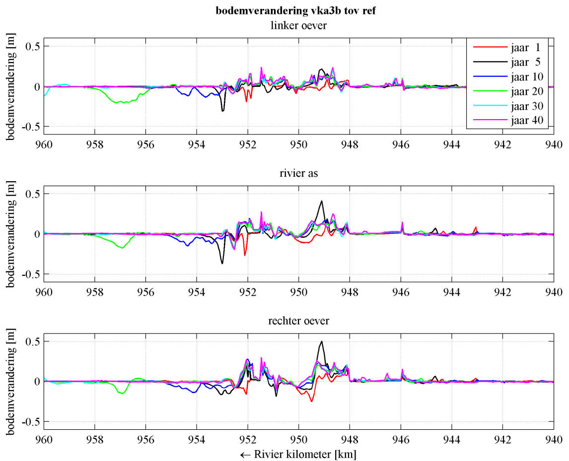
Figuur 3.2 Verskil in bodemniveau in een aantal jaar (na de laagwaterperiode) tussen ontwerpvariant VKA3b en de referentie voor simulaties zonder vaargeulbeheer langs (boven) de linkeroever, (midden) de as van de rivier en (beneden) de rechteroever.
