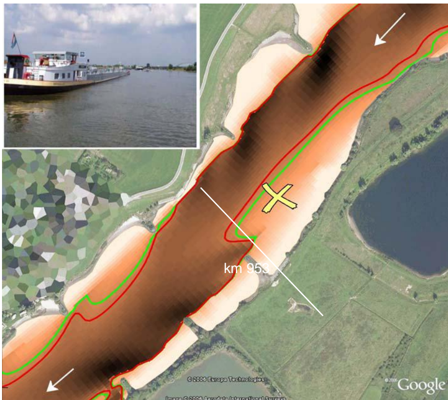
Figuur 3.4 Aanzanding ter plaatse van Klaphek (bron: Sloff, 2006).
