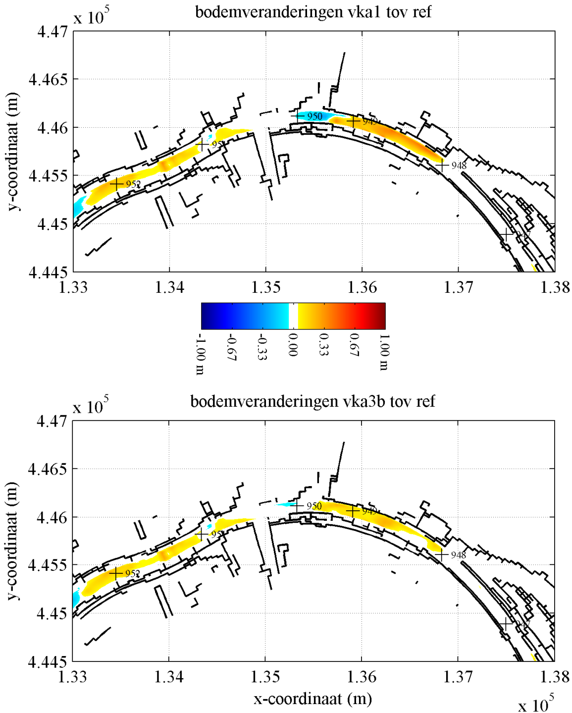
Figuur 3.1 (Vervolg) Verschil in bodemniveau in jaar 40 ter plaatse van het projectgebied voor simulaties zonder vaargeulbeheer na afloop van het laagwaterseizoen (na Q=209\text{m}^3/\text{s} ) (c) tussen ontwerpvariant VKA1 en de referentie, (d) tussen ontwerpvariant VKA3b en de referentie. De getallen duiden rivierkilometers aan.
