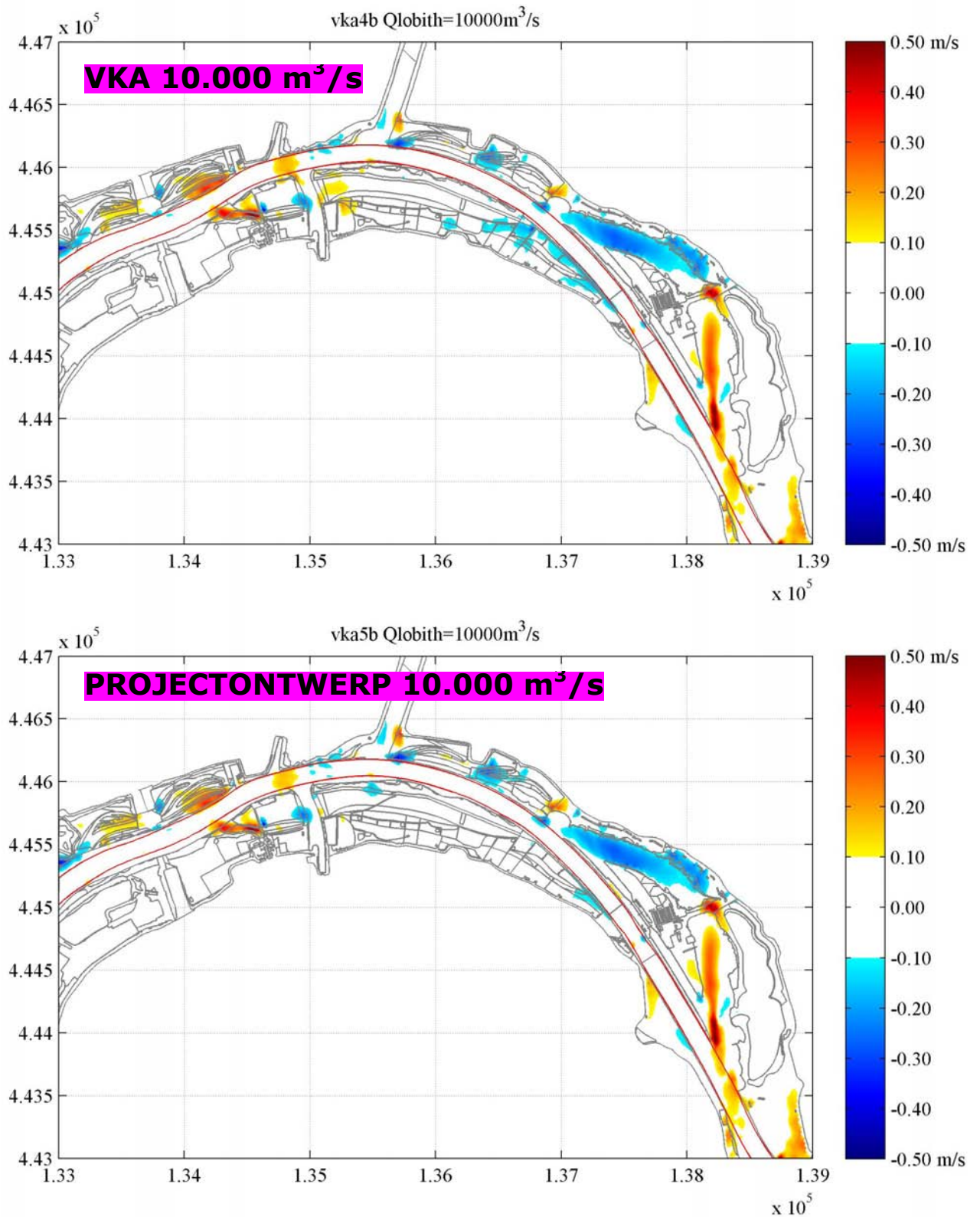
Figuur 23-2: Dwarsstromen bij 10.000 m 3 /s Lobith afvoer voor VKA (boven) en Projectontwerp (onder). In het onderste figuur is de kwelsloot in de Vianense Waard te herkennen. De kade ligt net ten noorden van deze kwelsloot.
