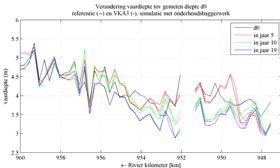
Figuur 3.13 Effect van de maatregelen op de gemiddelde diepte van de vaargeul voor simulaties met vaargeulbeheer en zonder zandwinning na het hoogwater; getrokken lijn: VKA3b, gestreepte lijn: referentie. d0 duidt een gemiddelde gemeten diepte aan (gemiddeld over vaargeul en vak van 250 m lengte), die is aangeleverd door J. Sieben.
