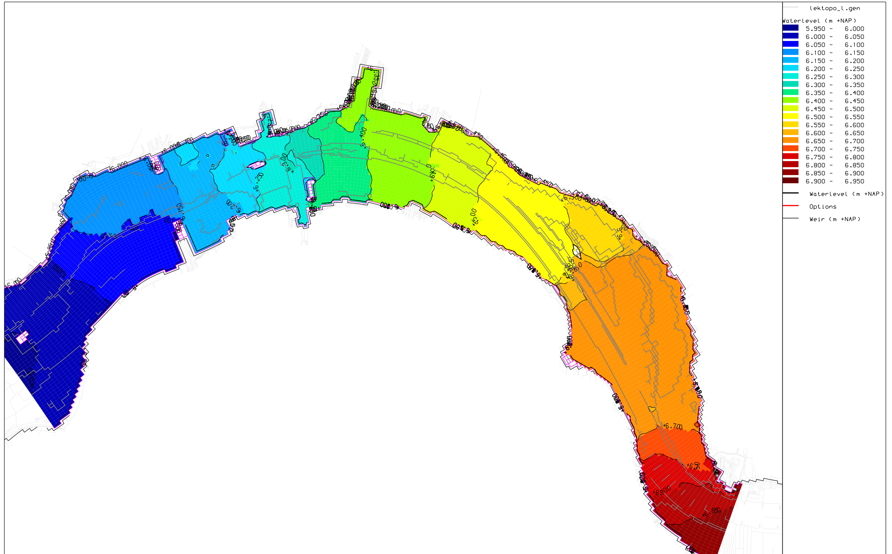
Vianen - VKA3a - interventieniveau Waterstanden bij Q Lobith = 16.000 m 3 /s
