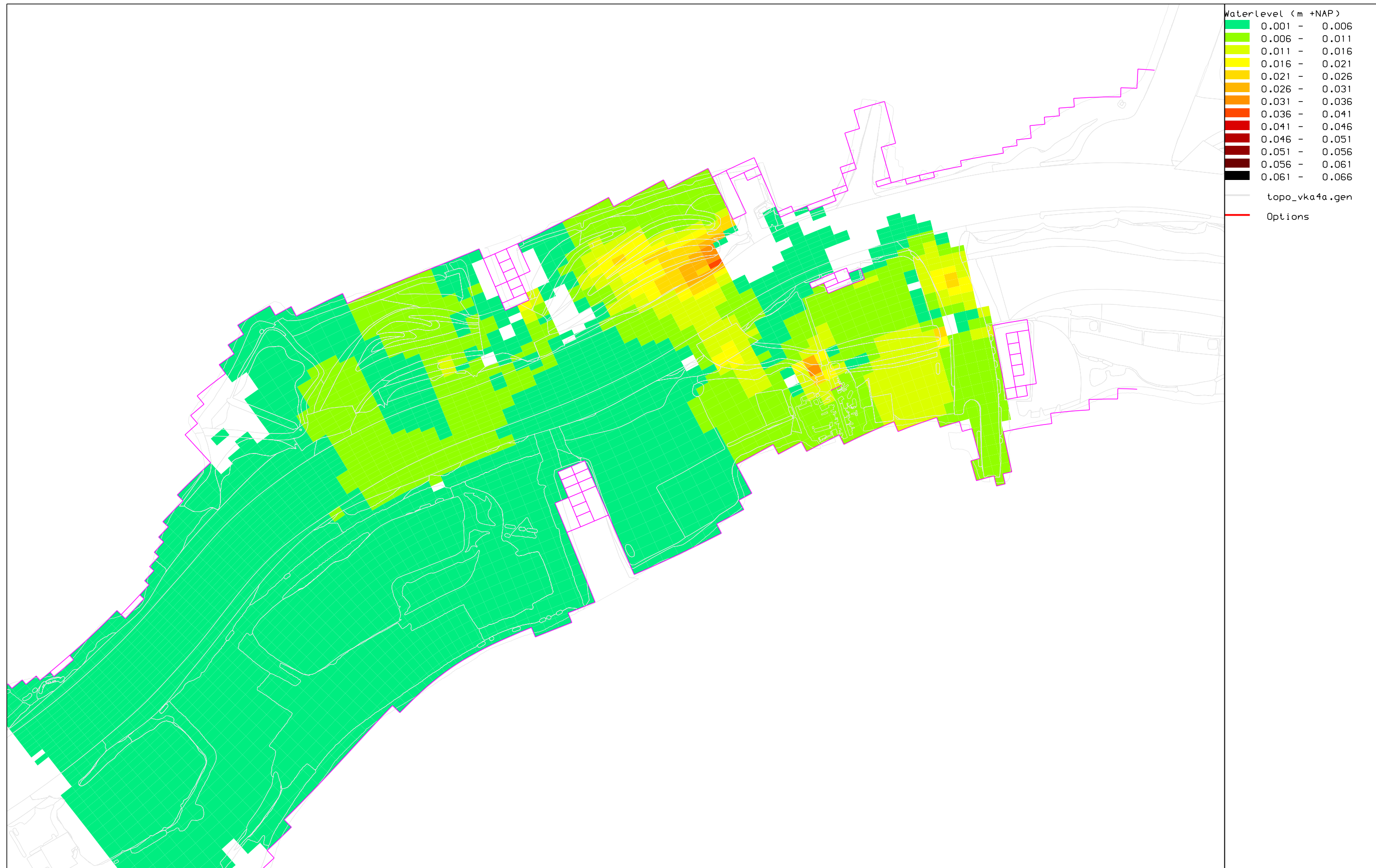
Ruimte voor de Lek Vianen - VKA - interventiebeeld (VKA4a) Waterstandsverhoging 2D t.o.v. referentie bij Q Lobith = 16.000 m 3 /s
