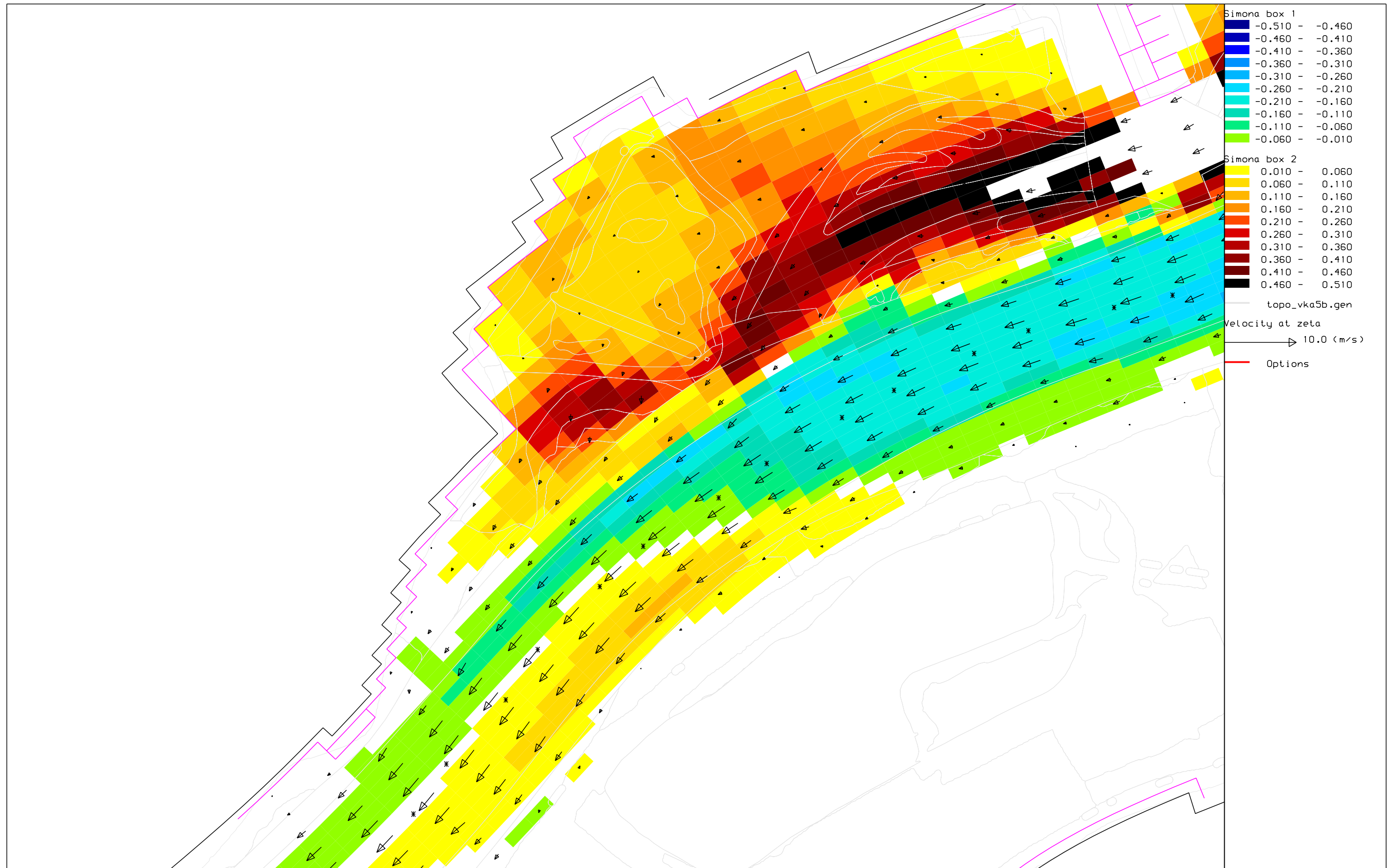
Vianen-Projectontwerp: verschil stroomsnelheid met referentie Verschil in m/s bij Q Lobith = 8.000 m 3 /s
