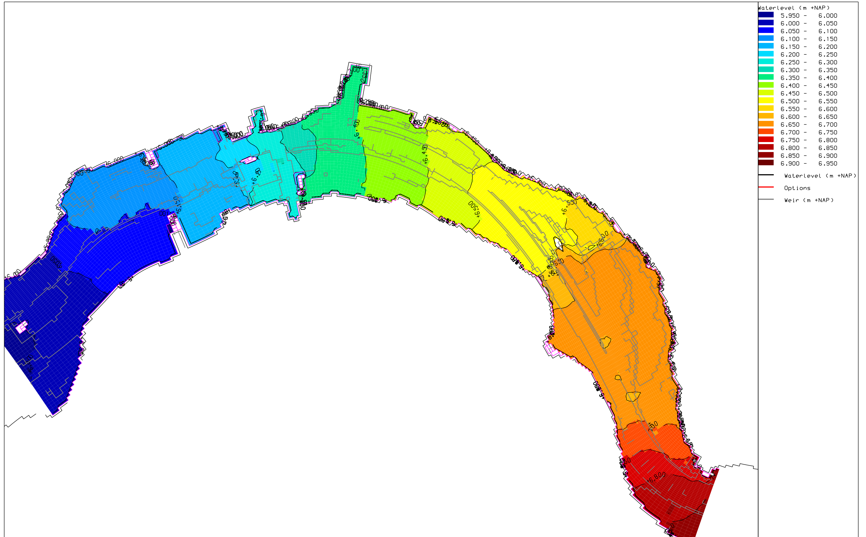
Vianen - VKA4 - streefbeeld Waterstanden bij Q Lobith = 16.000 m 3 /s
