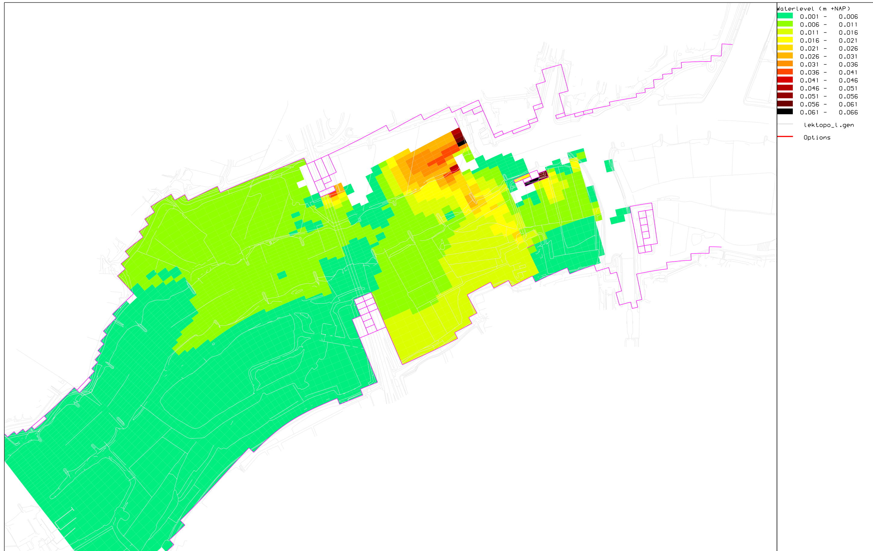
Ruimte voor de Lek Vianen - Gekozen Variant (SNIP2a) Waterstandsverhoging 2D t.o.v. referentie bij Q Lobith = 16.000 m 3 /s
