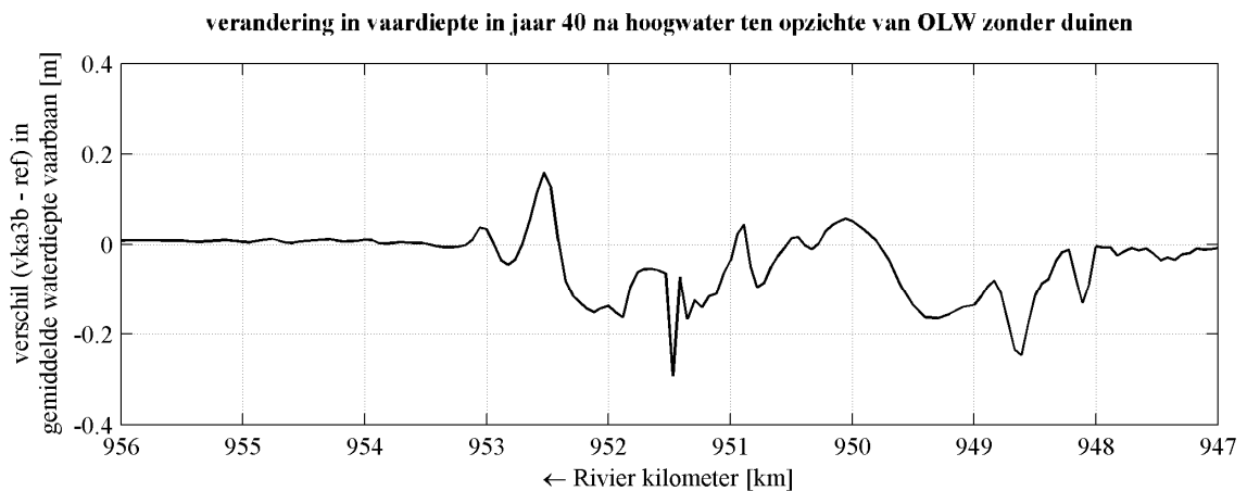
Figuur 3.7 Verschil tussen de gemiddelde diepte van de vaargeul ten opzichte van OLW in het VKA3b en de referentie na het hoogwater in jaar 40.
