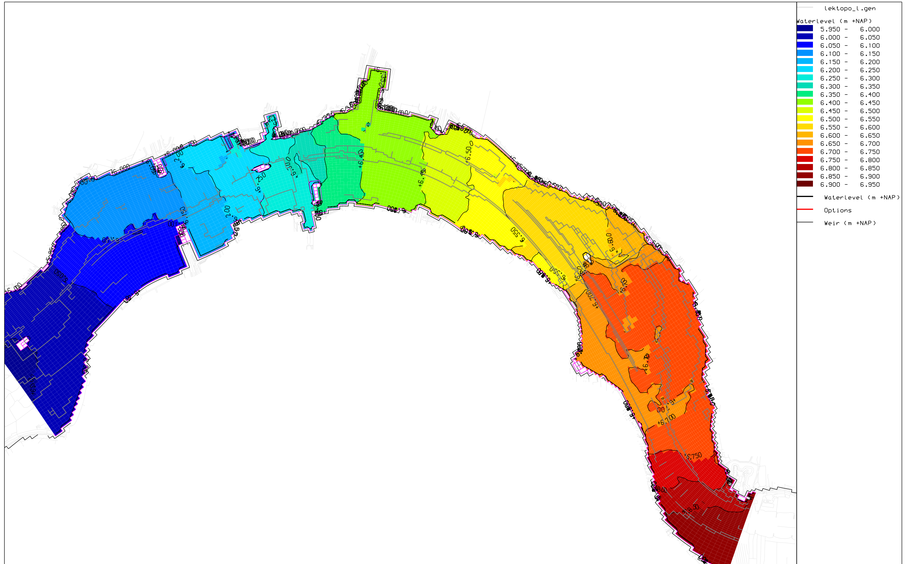
Vianen - VKA3c - doemscenario Waterstanden bij Q Lobith = 16.000 m 3 /s
