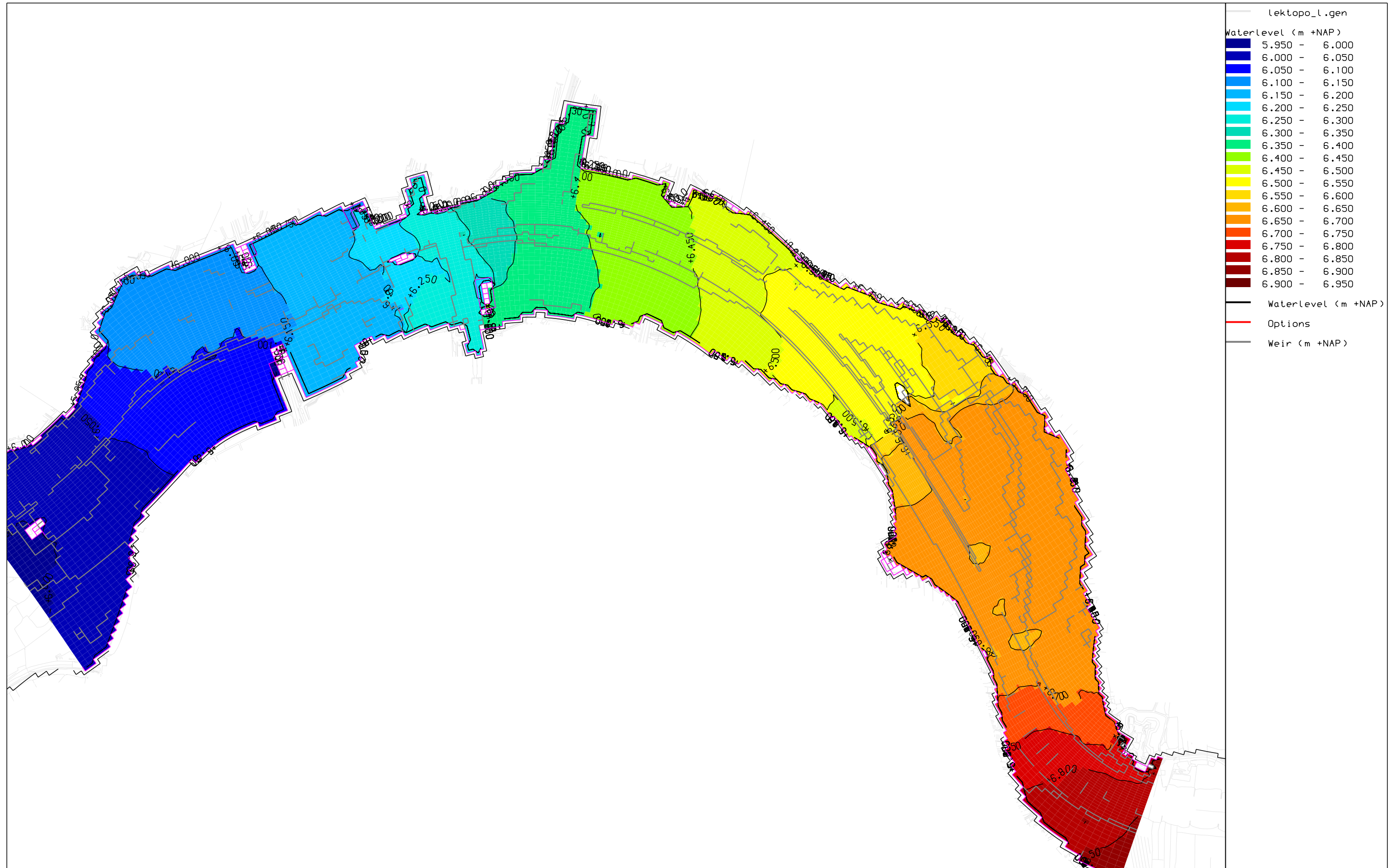
Vianen - VKA2b - streefbeeld Waterstanden bij Q Lobith = 16.000 m 3 /s
