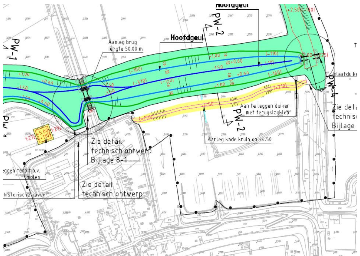
Figuur 11: Nieuwe kade Pontwaard.
