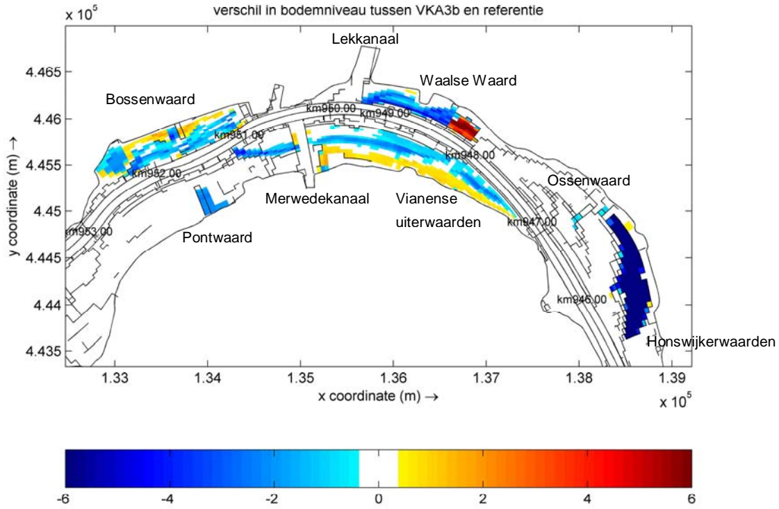
Figuur 2.1 Vershil in bodemniveau (in m) tussen ontwerpvariant en referentiesituatie op t = 0. De zwarte lijnen geven de normaallijnen, rivieras en overlaten voor de referentiesituatie weer.
