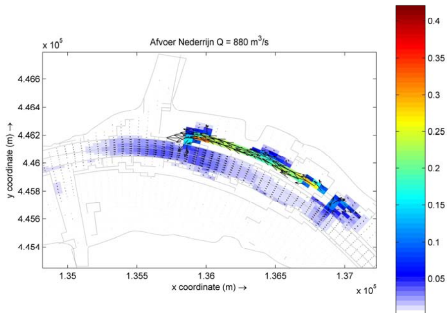
Figuur 9 Verschil in stroomsnelheid tussen voorkeursvariant en referentie bij 't Waalse waard voor afvoerniveau Q = 880 \text{ m}^3/\text{s} . De vectoren wijzen in de hoofdgeul richting oosten wat een afname in stroomsnelheid betekent ten opzichte van de referentie.
