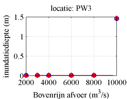
Figuur 7-5: Inundatiediepte Projectontwerp bij afvoeren variërend tussen 2.000 en 10.000 m 3 /s in uiterwaard ter plaatse punten in Figuur 7-1. Blauw: referentie, rood: Projectontwerp (streefbeeld)
