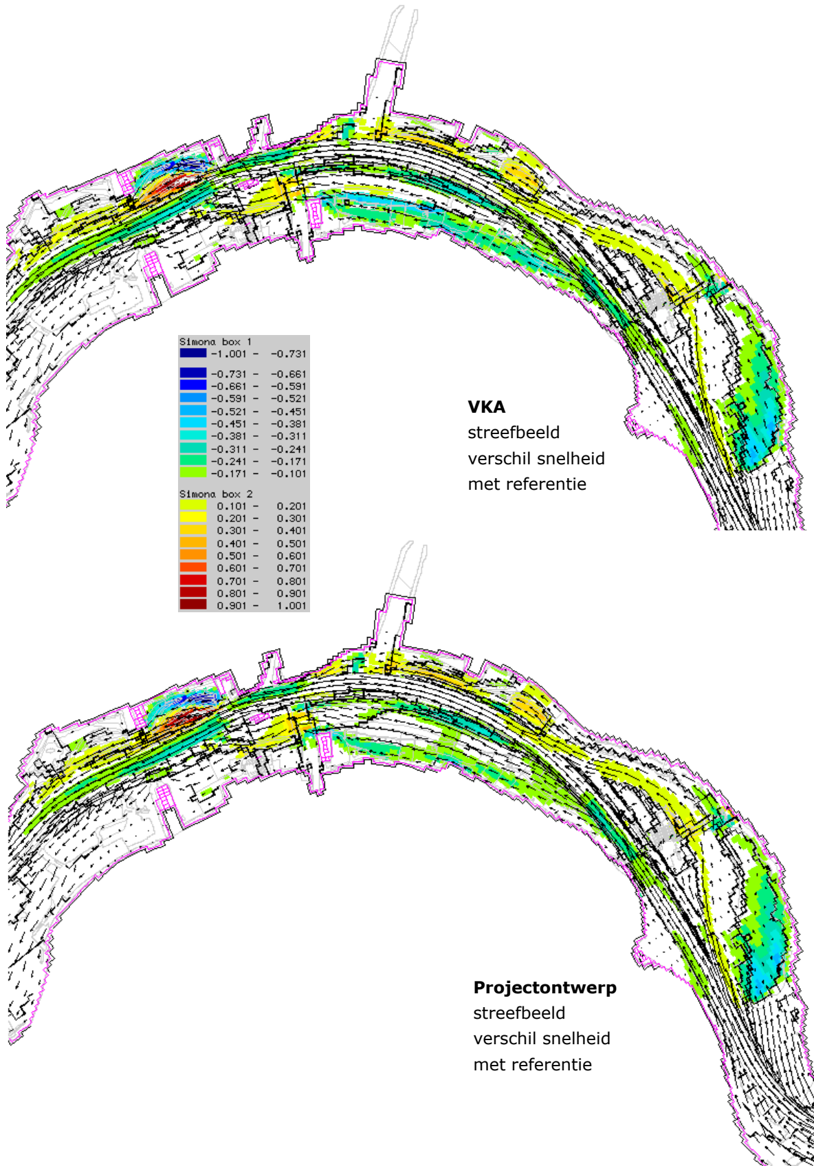
Figuur 6-8: Verschil in stroomsnelheid bij afvoer 16.000 m 3 /s met referentie voor VKA (boven) en Projectontwerp (onder). Negatieve waarden in de legenda betekenen een lagere stroomsnelheid; positieve waarden een vergroting. Verschillen kleiner dan 10 cm/s worden in dit figuur niet getoond. Vectors geven de snelheden na de ingreep. De overlaten zijn van na de ingreep.
