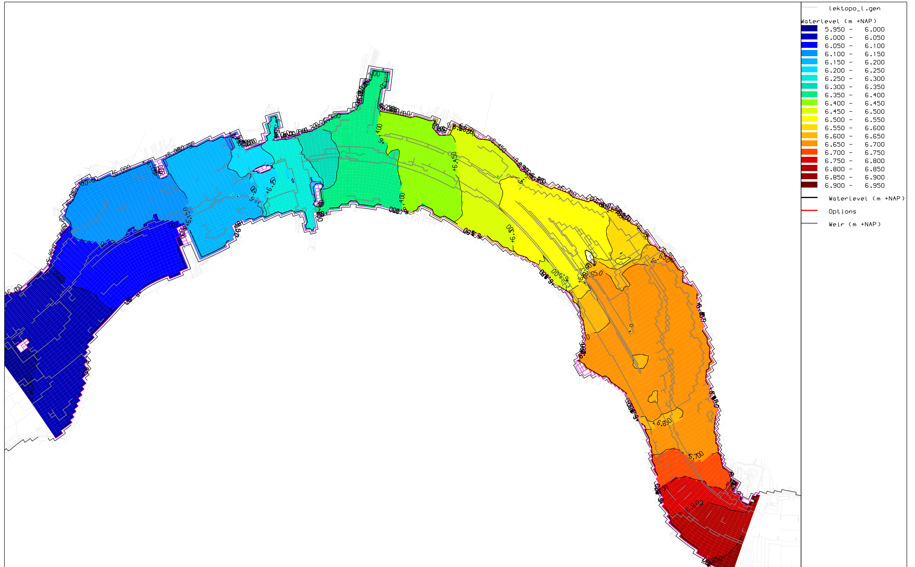
Vianen - VKA3b - streefbeeld Waterstanden bij Q Lobith = 16.000 m 3 /s
