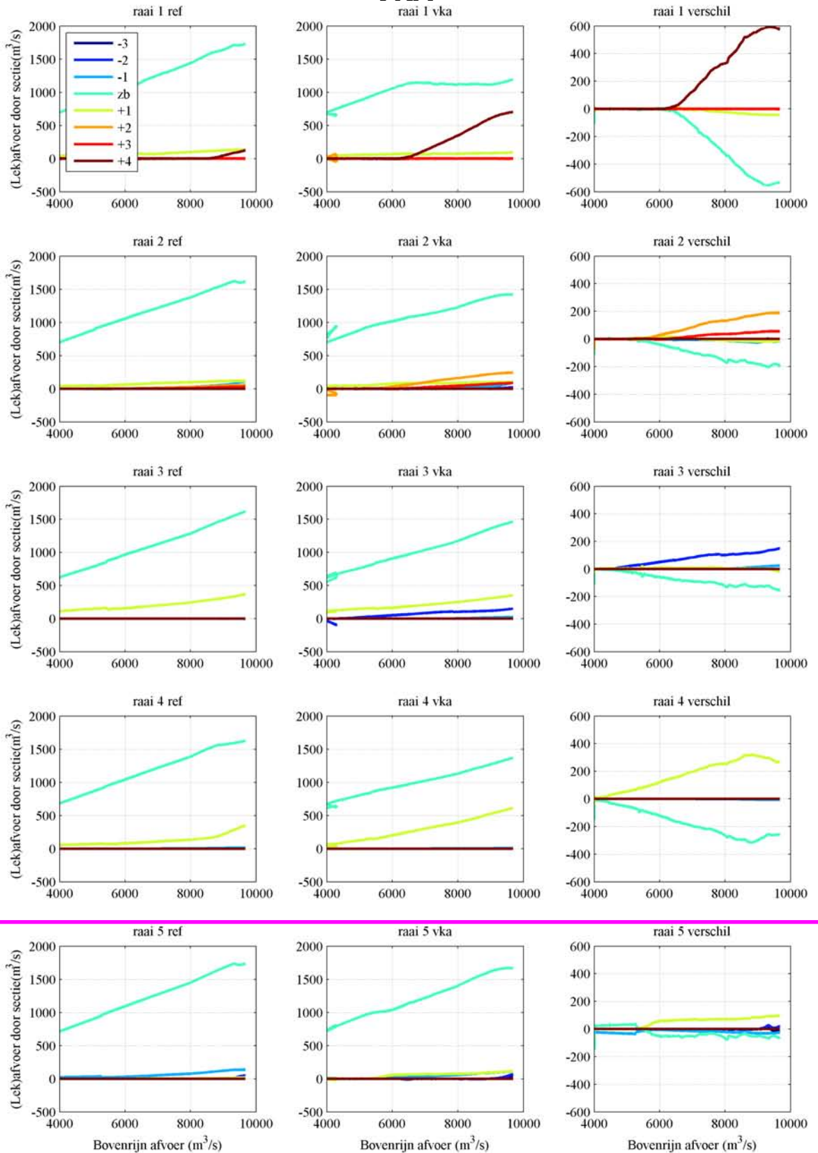
Figuur 7-2: Afvoerverdeling zomerbed en uiterwaardsecties voor 5 dwarsraaien. Linker panelen: referentie, midden panelen: VKA met streefbeeld ruwheden en bodemligging, rechter panelen: verschil (VKA minus referentie). De legenda geeft de opsplitsing van de raaien weer: zb=zomerbed secties, -1 betekent eerste sectie op linker oever, -2 betekent tweede sectie op linker oever, etc.
