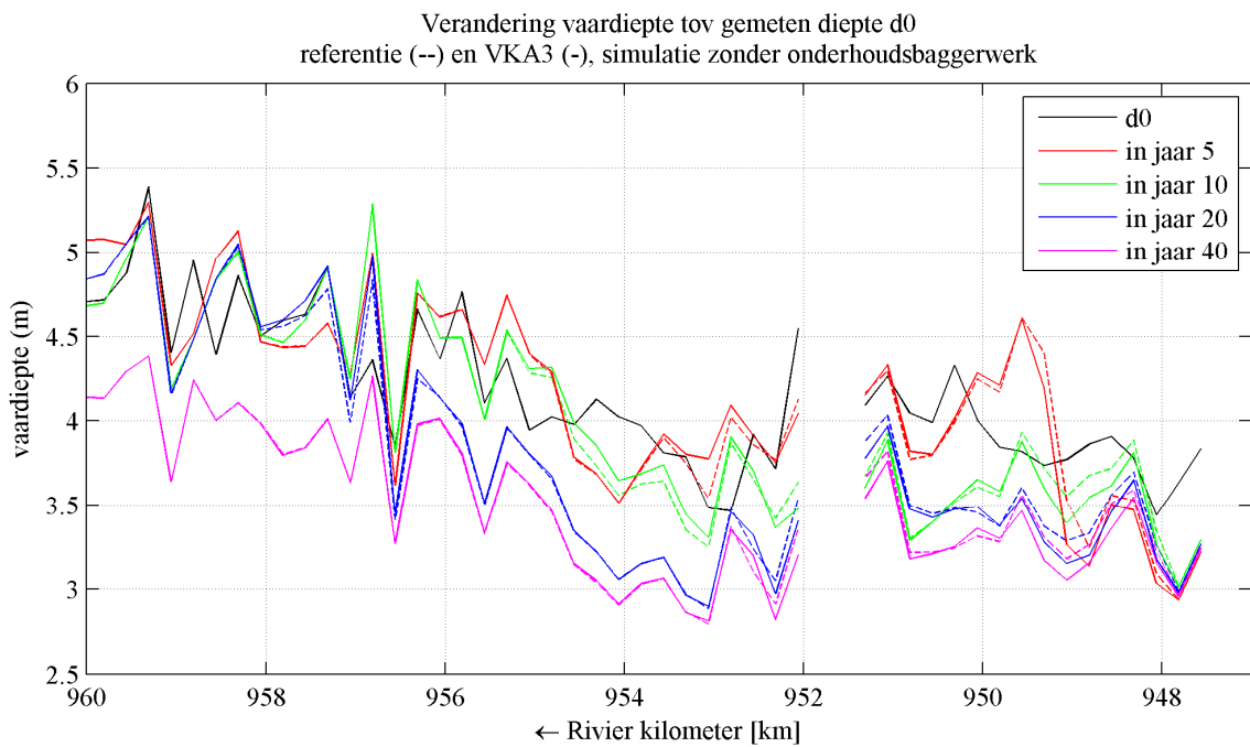
Figuur 3.6 Effect van de maatregelen op de gemiddelde diepte van de vaargeul voor simulaties zonder vaargeulbeheer na het hoogwater; getrokken lijn: VKA3b, gestreepte lijn: referentie. d0 duidt een gemiddelde gemeten diepte aan (gemiddeld over vaargeul en vak van 250 m lengte), die is aangeleverd door J. Sieben.
