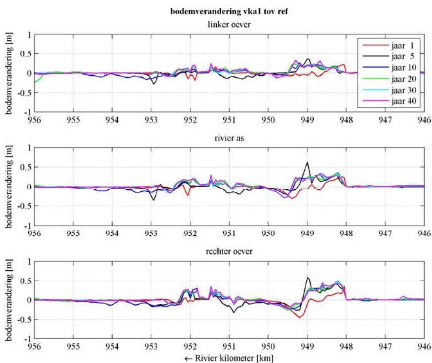
Figuur 4 Verschil in bodemniveau na een aantal jaren tussen ontwerpvariant VKA1 en de referentie langs (boven) de linkeroever, (midden) de as van de rivier en (beneden) de rechteroever. Figuur gemaakt door HKV.
