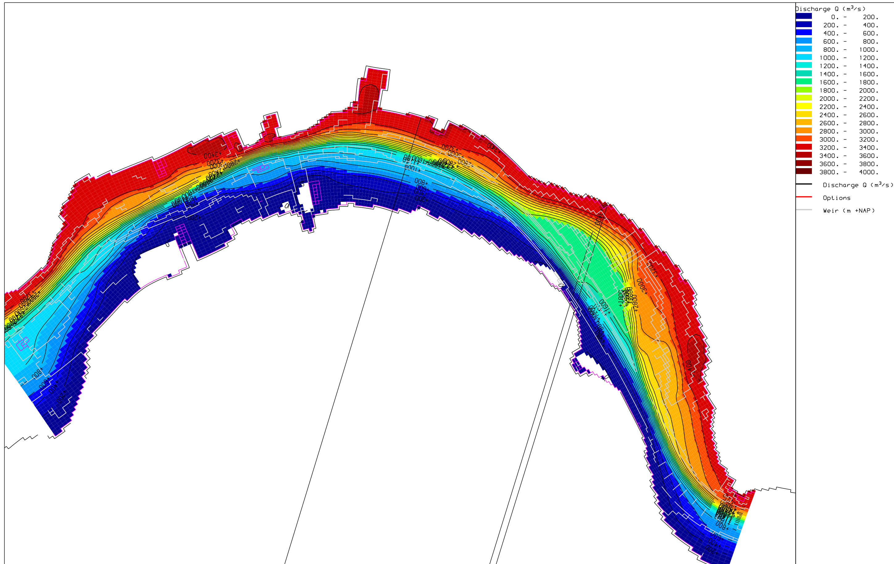
Vianen - VKA3a - interventieniveau Afvoerlijnen bij Q Lobith = 16.000 \text{m}^3/\text{s}
