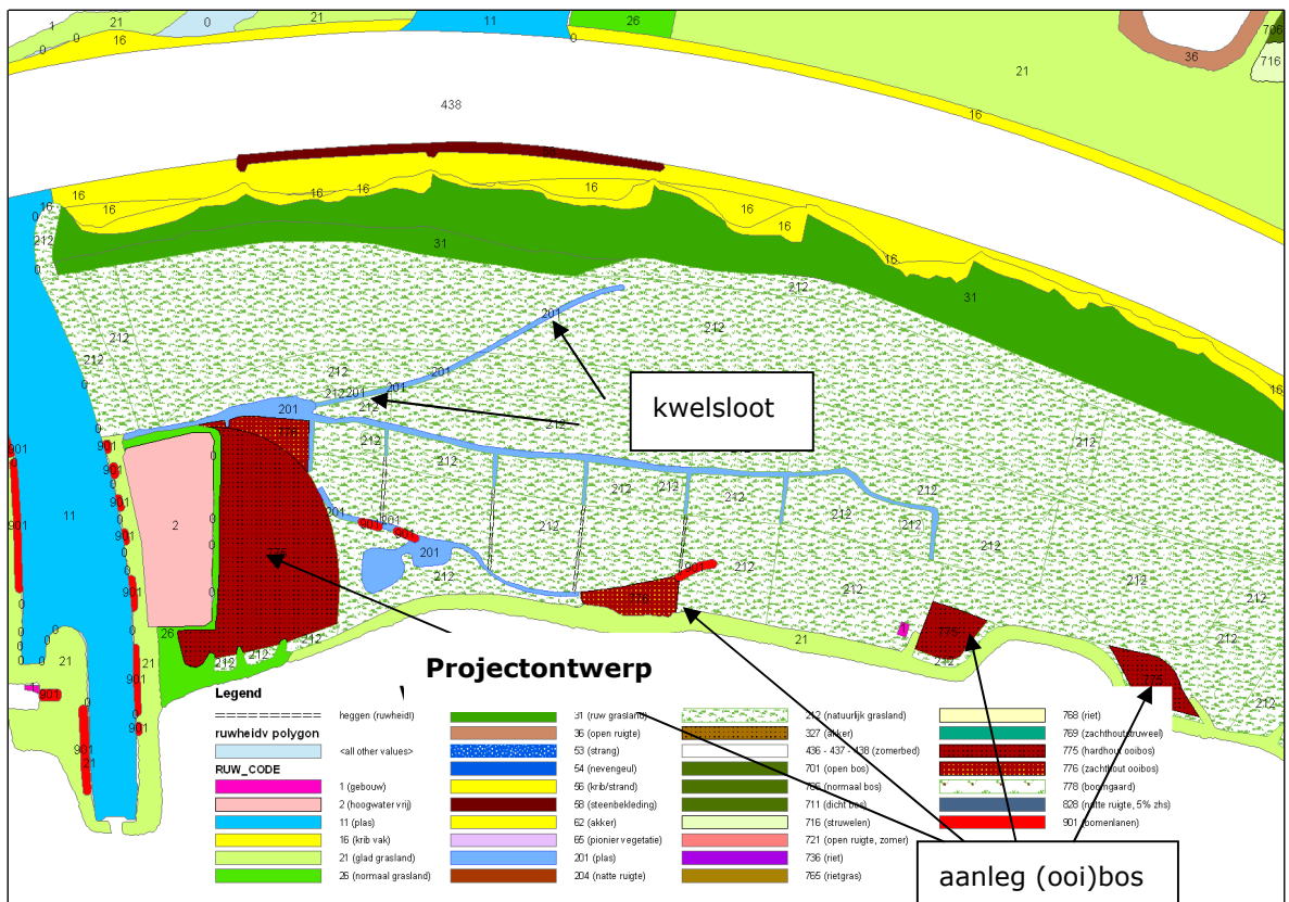
Figuur 4-4: Ruwheidsvlakken in huidige situatie (boven) en Projectontwerp (onder).
