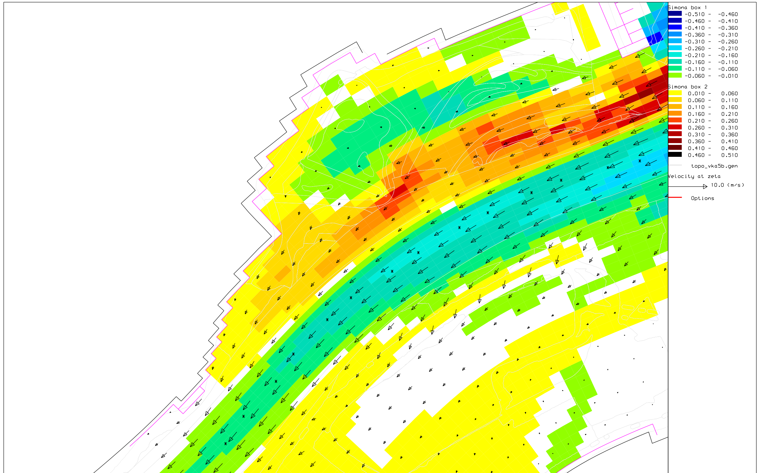
Vianen-Projectontwerp: verschil stroomsnelheid met referentie Verschil in m/s bij Q Lobith = 16.000 m 3 /s
