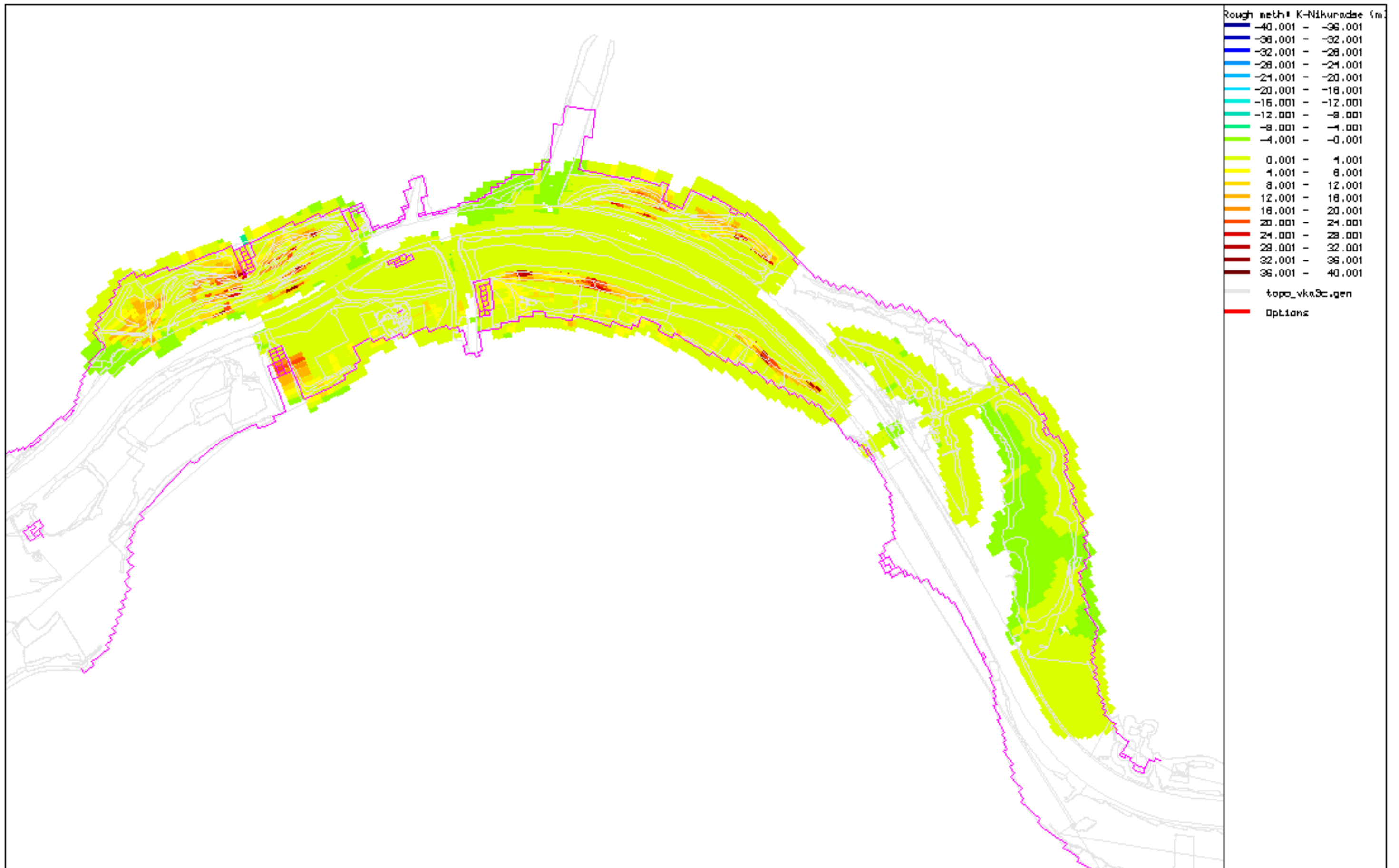
Vianen - VKA3a - interventieniveau Verschillen ruwheidshoogte t.o.v. referentie Nikuradse k in m
