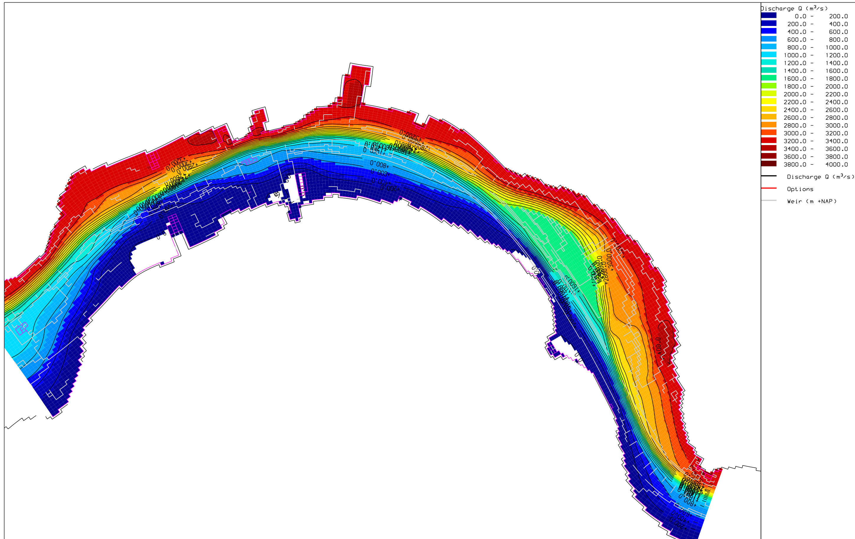
Vianen - VKA2a - doemscenario Afvoerlijnen bij Q Lobith = 16.000 m 3 /s
